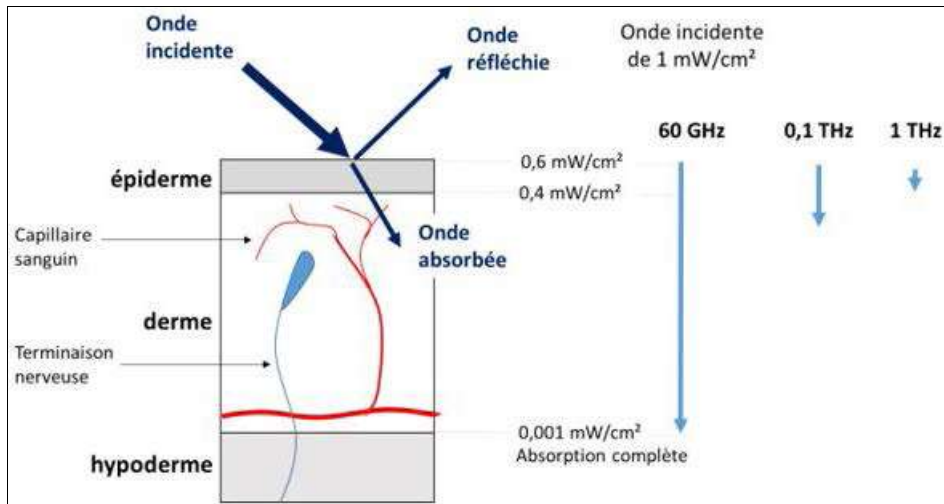
Figure 6 : Pénétration d'un rayonnement électromagnétique de type radiofréquences dans le corps humain en fonction de la fréquence
