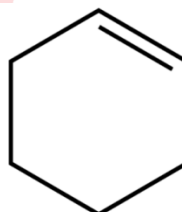
ciclohexeno
