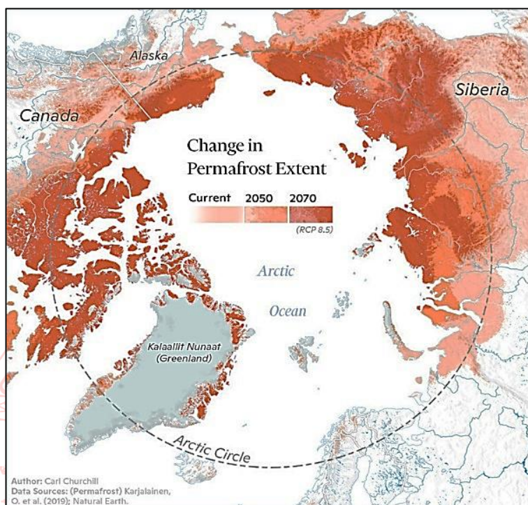
Reducción del permafrost en el Ártico
