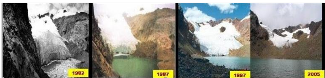
Glaciar Yanamarey – Cordillera Blanca – 4 890 m s. n. m. (1 982 – 2 005)
