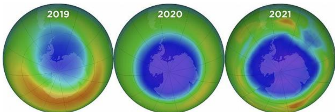
Evolución del agujero de la capa de ozono desde 2019 al 2021
