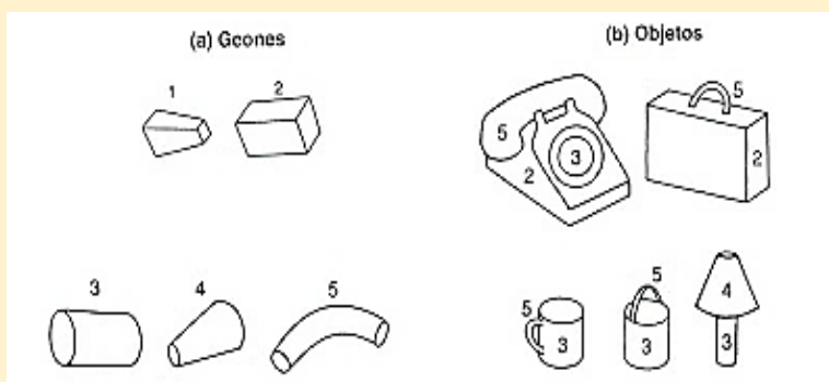
Fig. 7-6. Teoría de geones de Biederman.
