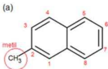
2 – metilnaftaleno β – metilnaftaleno
