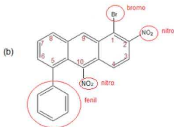
1–bromo – 5 – fenil – 2,10 – dinitroantraceno α – bromo – α – fenil – β,γ – dinitroantraceno
