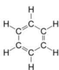
benceno : C_6H_6
