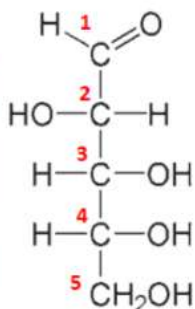
2,3,4,5 – tetrahidroxipentanal
