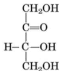
Eritrulosa
