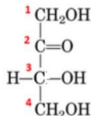
1,3,4 – trihidroxibutan – 2 – ona
