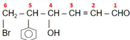
6 – bromo – 5 – fenil – 4 – hidroxihex – 2 – enal
