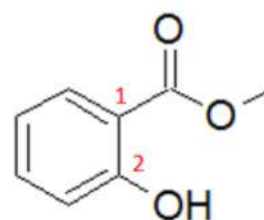
2 – hidroxibenzoato de metilo
