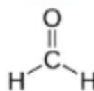
Metanal
