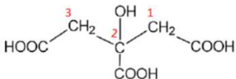
Ácido 2 – hidroxipropano – 1,2,3 – tricarboxílico
