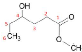
4 – hidroxihexanoato de metilo
