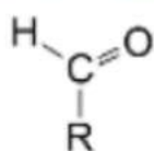
Aldehído
