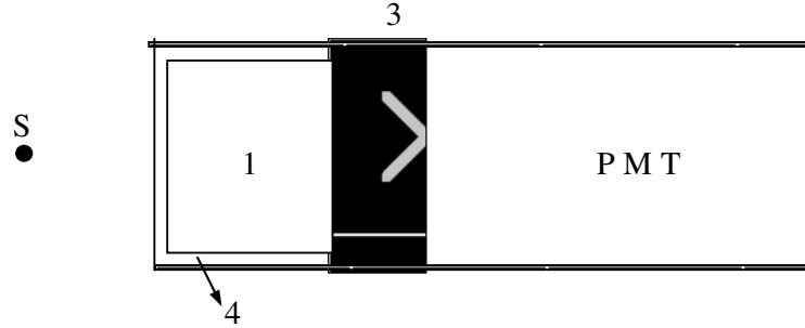
شكل (4-16): الكاشف الومضي
