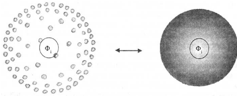
Рис. 19. Любой объект ( \Phi_i ) — это пора в эфире. Он окружен эфирными слоями, в которых плотность максимума по мере удаления от объекта растет, пока не достигает предельной теоретической на очень удаленном (возможно, бесконечном) расстоянии от объекта.
