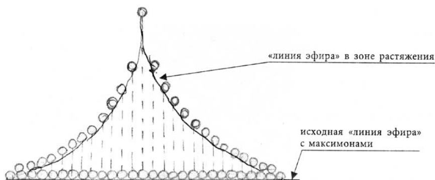
Рис. 28. Очевидно, что плотность максимонов падает по мере приближения к возмущённой зоне эфира.
