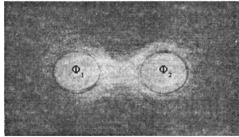
Рис. 25. Два тела \Phi_1 и \Phi_2 с эфирными слоями разрезания вокруг них.
