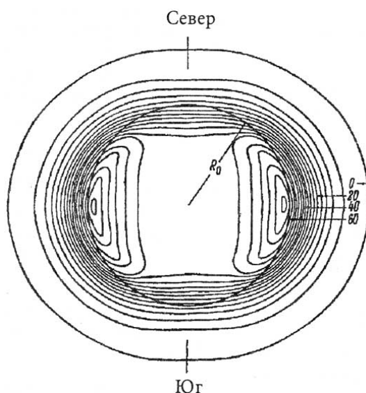
Рис 33. Двумерное распределение радиояркости по диску Солнца на волне 21 см. Линии проведены через одинаковые интервалы температуры в 4000 К. Яркостная температура в центре 47 000 К, а максимальной яркости соответствует температура 68 000 К. (Кристиансен и Варбургтон.)
