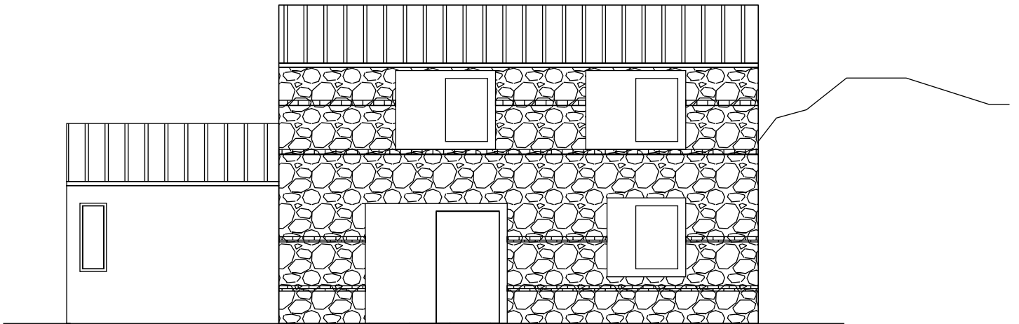
Prospetto frontale
