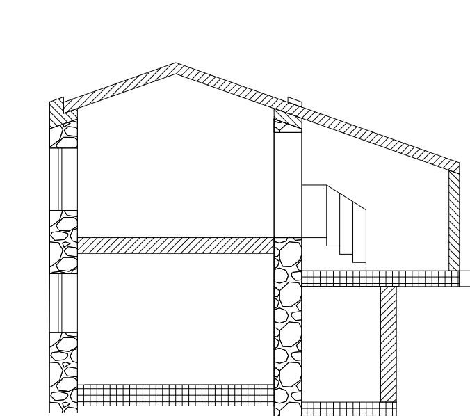
Sezione A-A
