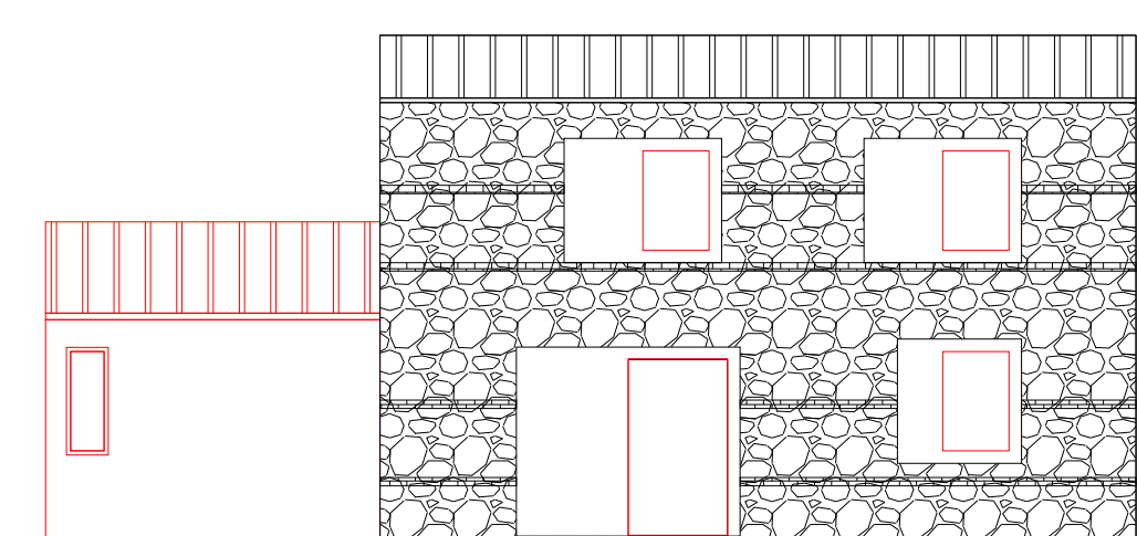
Prospetto Frontale
