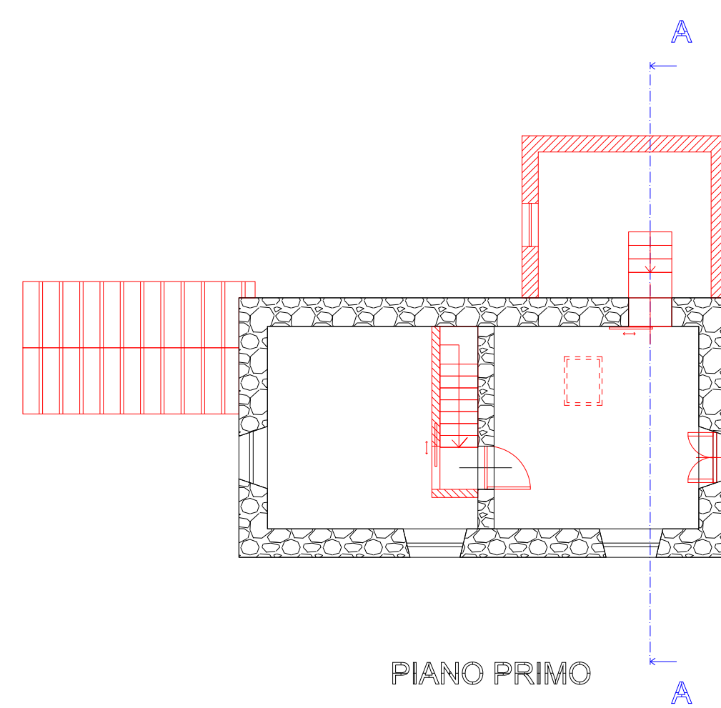
PIANO PRIMO
