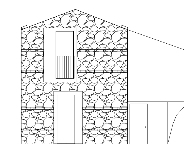
Prospetto Lato Destra
