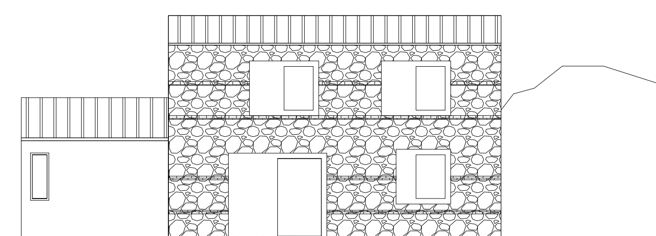
Prospetto Frontale
