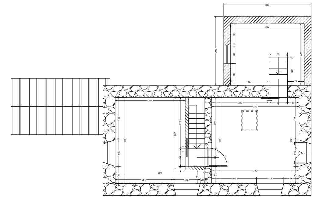
PIANO PRIMO
