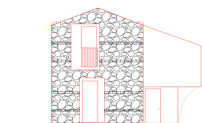
Prospetto Lato Destra
