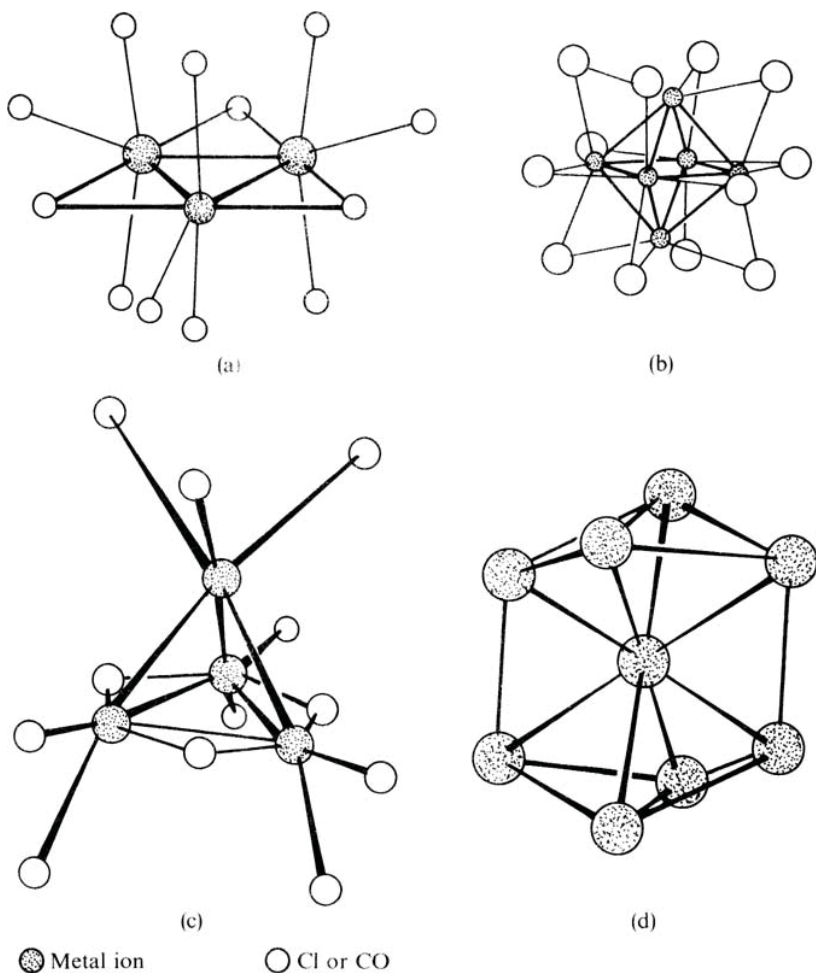
Figure 3.3 Structures of metal clusters, (a) \text{Re}_3\text{Cl}_{12}^{3-} ; (b) \text{Rh}_6(\text{CO})_{12} ; (c) \text{Co}_4(\text{CO})_{12} ; (d) \text{AuAu}_8 in [\text{AuAu}_8(\text{PPH}_3)_8]^{3+} .
