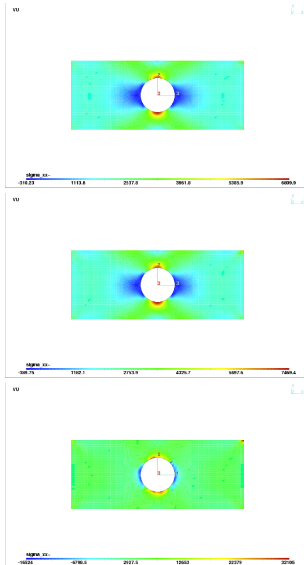
Figure 10.7 – Contrainte \sigma_{11} : \nu = 0,3 , \nu = 0,4 et \nu = 0,4999
