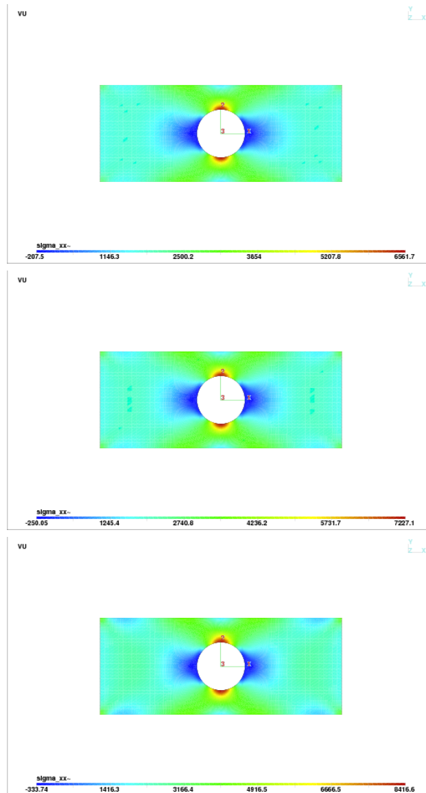
Figure 12.3 – Contrainte \sigma_{11} : \nu = 0,3 , \nu = 0,4 et \nu = 0,4999
