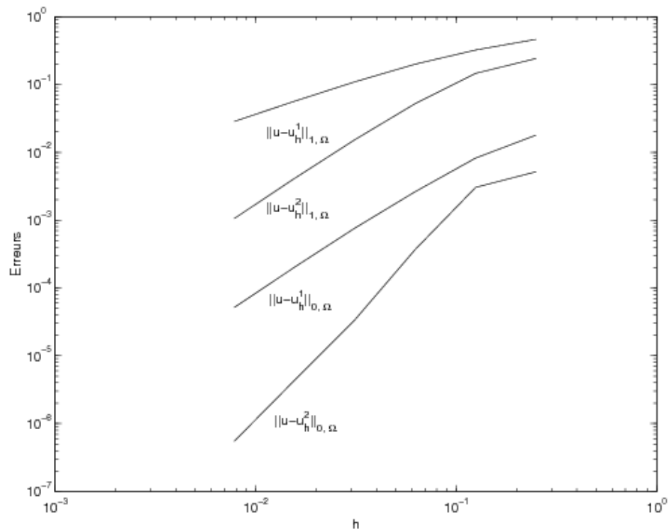
Figure 7.2 – Erreurs commises pour les approximations linéaire et quadratique
