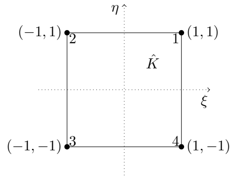
Figure 6.4 – Élément de référence quadrangulaire à 4 noeuds ( n_g^K = 4 )
