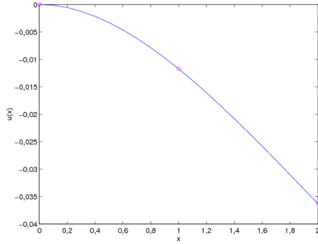
Figure 5.16 – Déformation de la poutre encastrée
