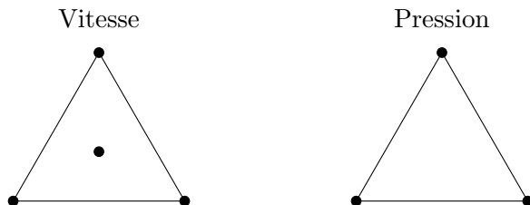
Figure 11.1 – Élément Mini ( O(h) )
