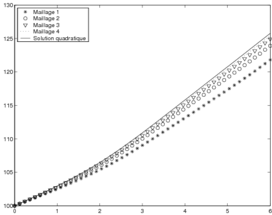
Figure 7.5 – Coupe de la température sur l'axe y = 1
