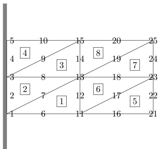
Figure 10.1 – Maillage, numéros d'éléments et numéros noeuds de calcul
