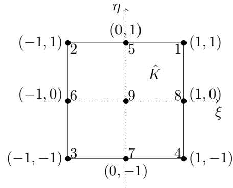
Figure 6.5 – Élément de référence quadrangulaire à 9 noeuds ( n_g^K = 9 )
