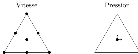
Figure 11.10 – Élément à pression discontinue de Crouzeix-Raviart P_2^+ - P_1 ( O(h^2) )
