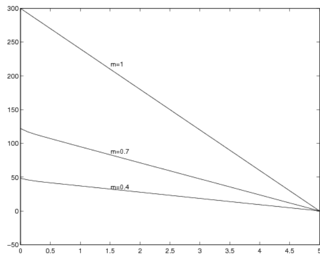
Figure 11.19 – Perte de charge dans le canal
