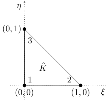
Figure 6.2 – Élément de référence triangulaire à 3 noeuds ( n_g^K = 3 )
