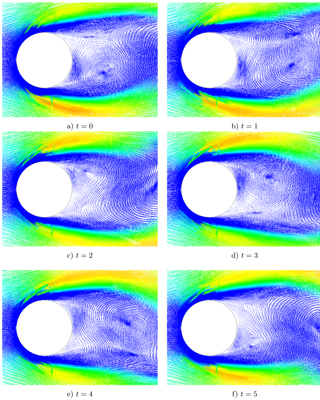
Figure 11.24 – Champ de vitesse derrière le cylindre à Re = 100 sur une période
