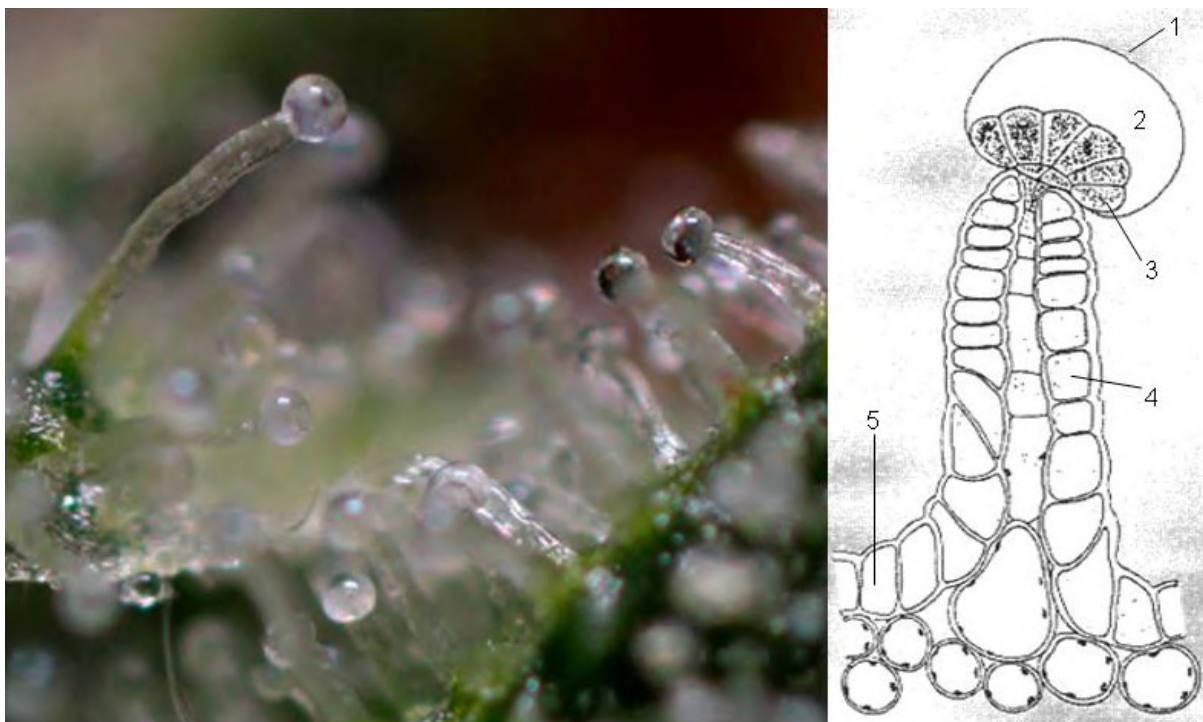
Figuur I-1 Elektronenmicroscopische opname van de harskliertjes, de trichomen, van de cannabisplant (Bron: www.THCFarmer.com). Rechts schematische weergave van een trichoom (Bron: Briosi en Tognini, 1894). 1 = waslaag; 2 = excretieruimte; 3 = kliercellen; 4 = halscellen; 5 = epidermiscellen.
