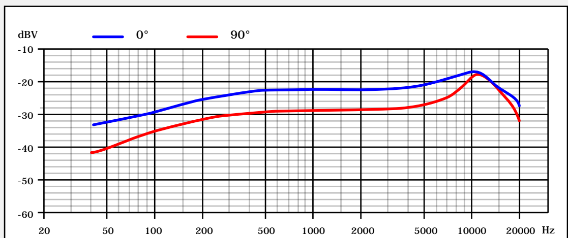
Respuesta en frecuencia de una capsula Sennheiser ME104
